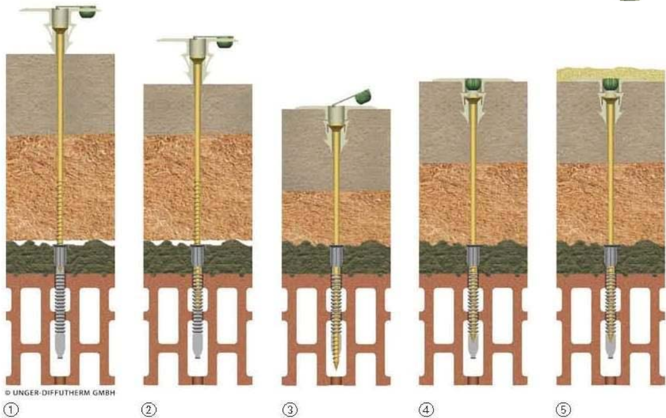
① Nach Vorbohren Dübel setzen ② Dübel bis Anschlag einschrauben ③ Einschrauben, bis Rückholverschluss einrastet und sich Dübelkopf in oberer Dämmebene verkrallt ④ Dübel nach Wasserwaage oder Laser justieren ⑤ Nach kompletter Dämmmontage erfolgt der Putzaufbau
