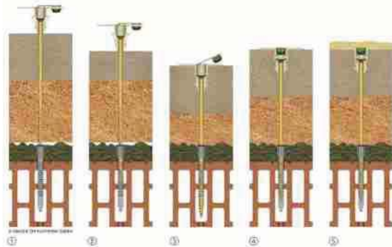
Das geniale Reco-Prinzip funktioniert mit patentiertem Stelldübel inklusive Rückstellfunktion
